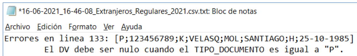
Imagen 12: Archivo de texto con los errores encontrados identificado con su número de línea.
